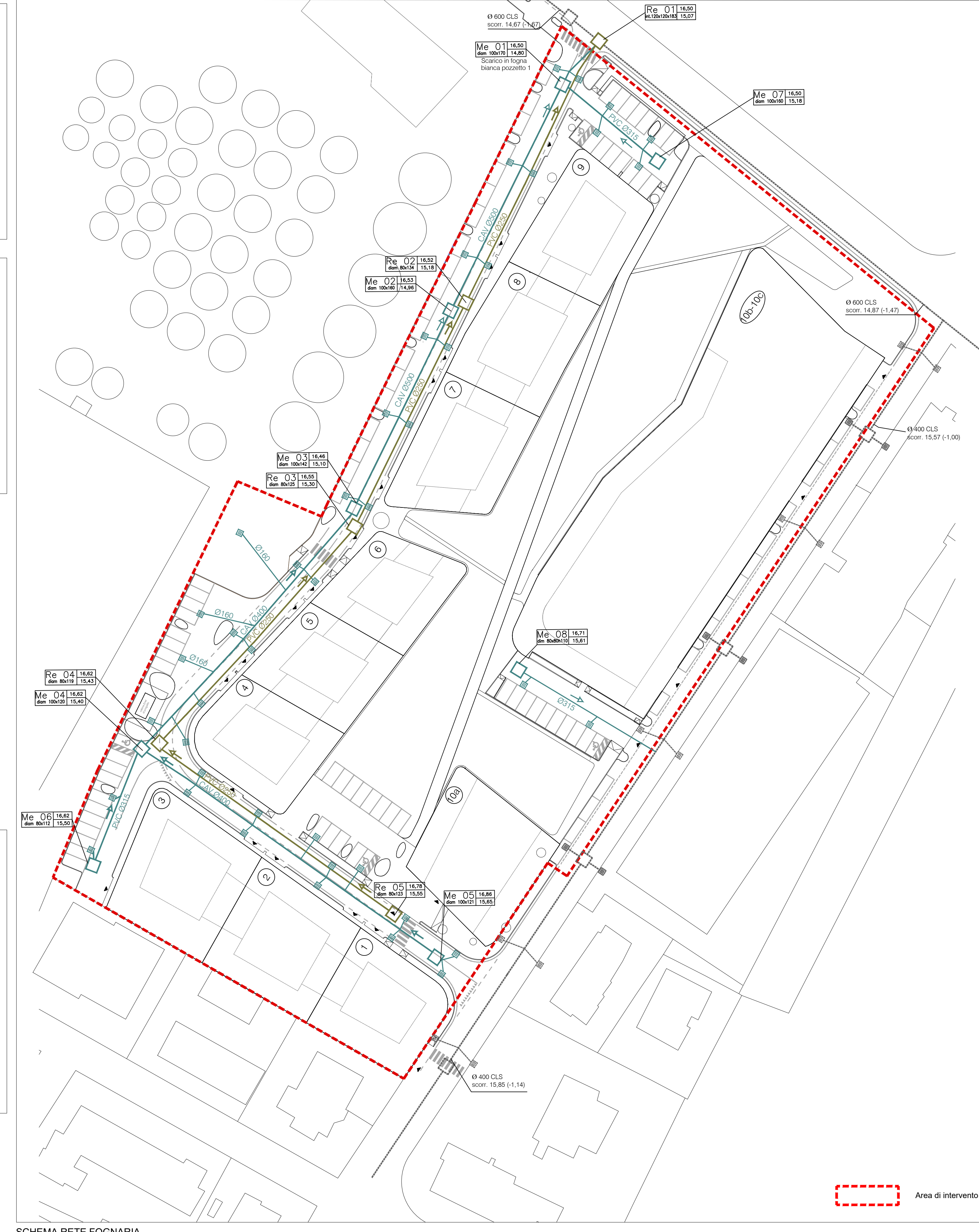
SCHEMA RETE FOGNARIA
