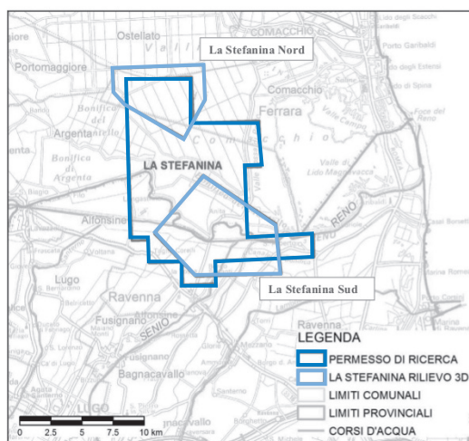
Inquadramento Territoriale del Permesso di Ricerca e delle Aree Rilievo Geofisico 3D La Stefanina (CTR 1:250,000 Regione Emilia Romagna)
