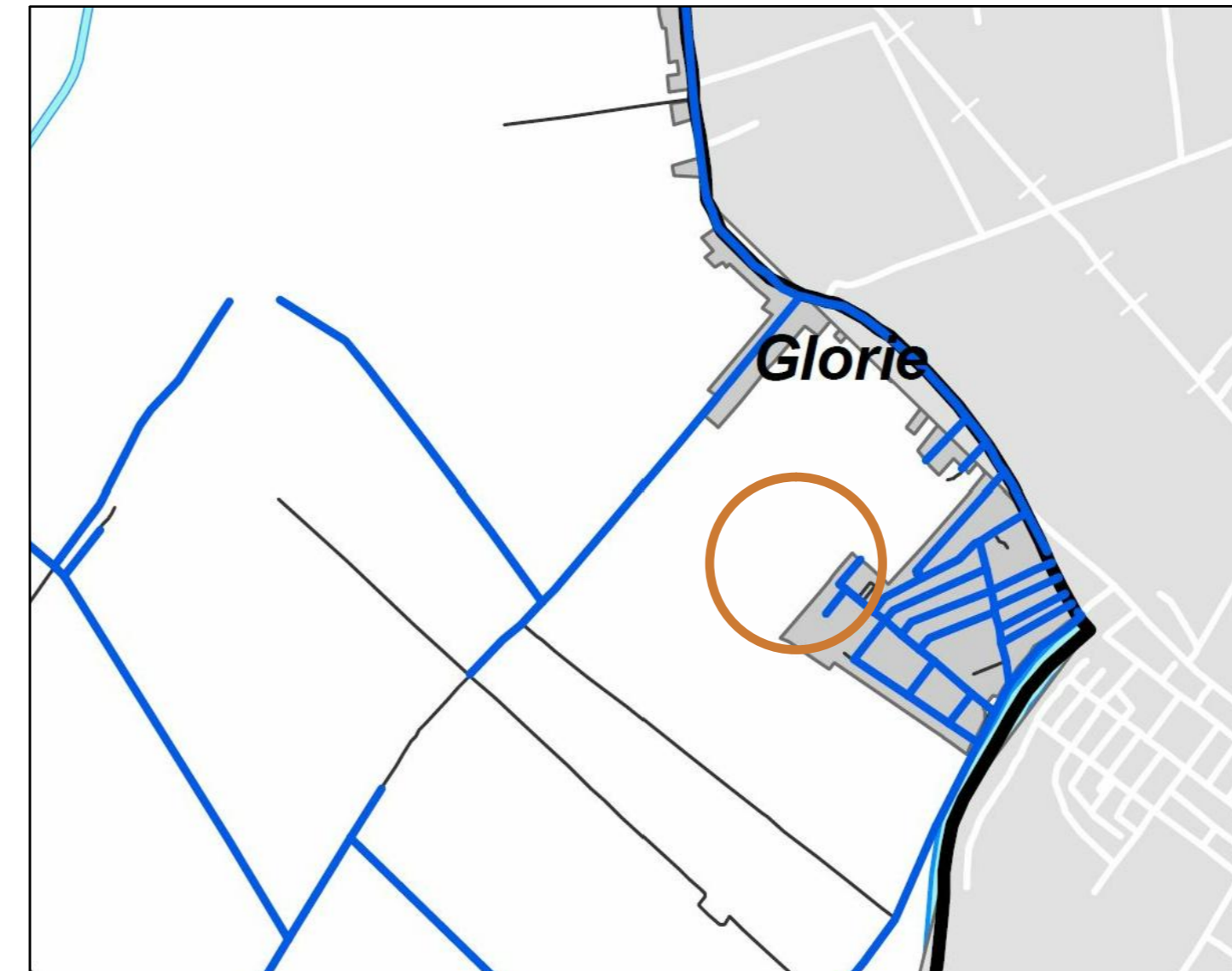
RETE IDRICA: Quadro conoscitivo Tav.7 Rete distribuzione idrica
